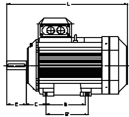
Foot mounted motor IM 1001 / B3
